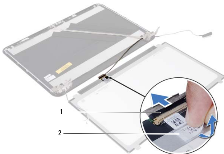
1 beeldschermkabel 2 tape
